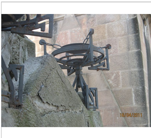
Detall element forja AS-DB
