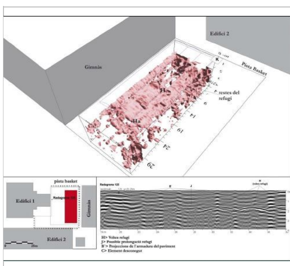
Refugi número 1-Restitució planimètrica MHS
