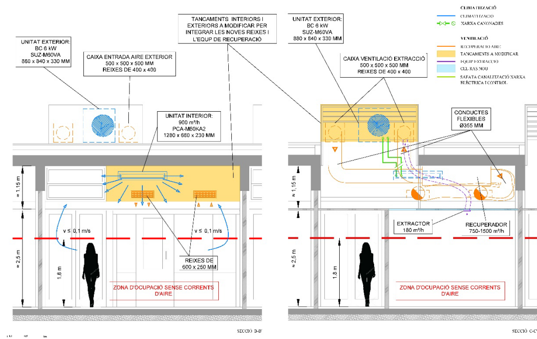
SECCIONS TRANSVERSALS AULA TIPUS
