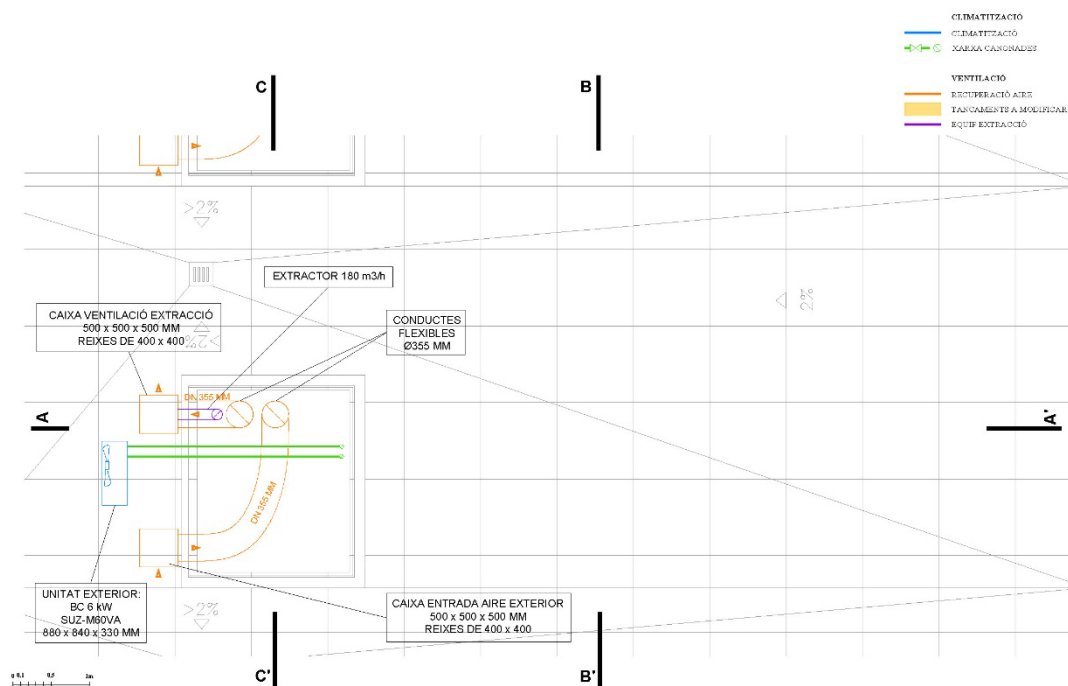
PLANTA COBERTA AULA TIPUS
