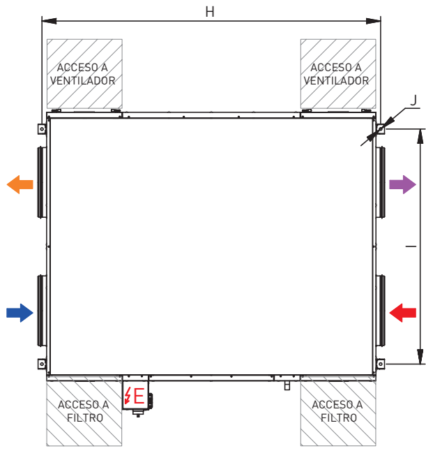
CONFIGURACION RESULTADO DE SIMPLE MODIFICACIÓN EN OBRA
