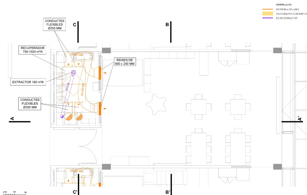
PLANTA AULA TIPUS
