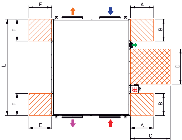
VISTA SUPERIOR POR DEFECTO (SUMINISTRO DE FÁBRICA)
