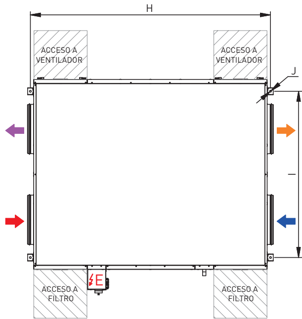
POR DEFECTO (SUMINISTRO DE FÁBRICA)
