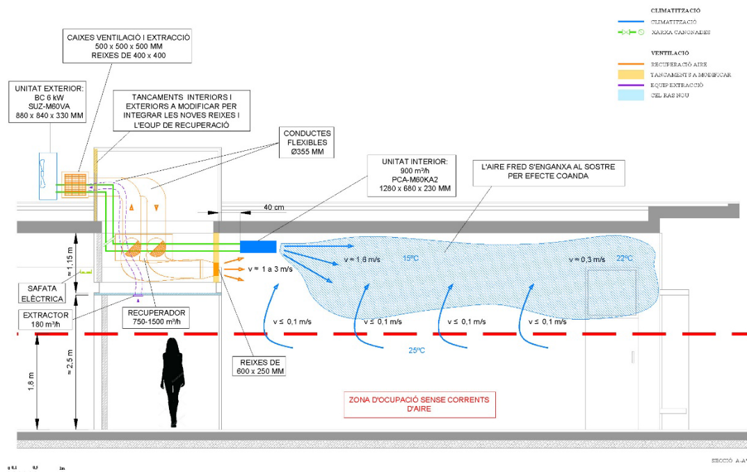
SECCIÓ LONGITUDINAL AULA TIPUS
