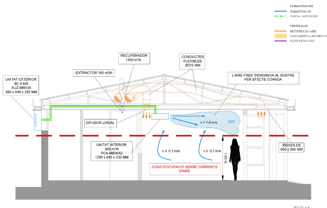
SECCIÓ LONGITUDINAL AULA TIPUS
