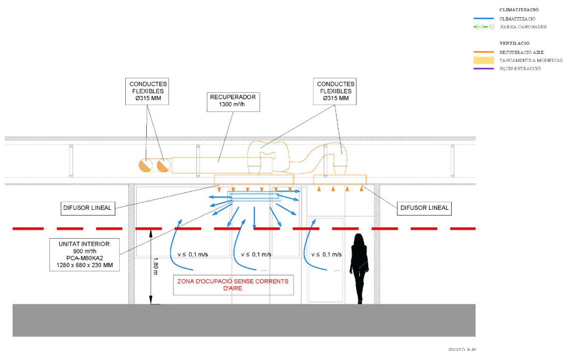
SECCIÓ TRANSVERSAL AULA TIPUS
