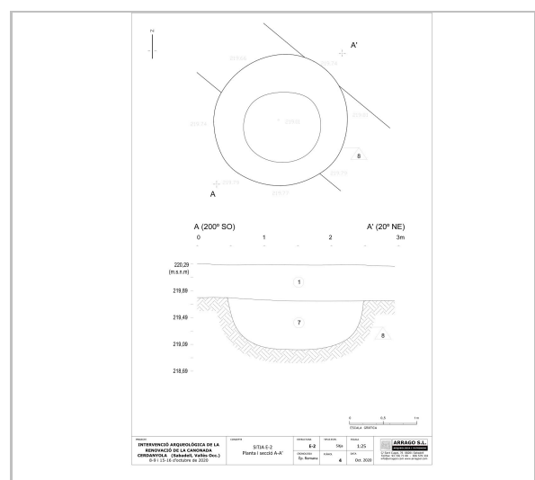
Planta i secció sitja E-2 ARRAGO SL
