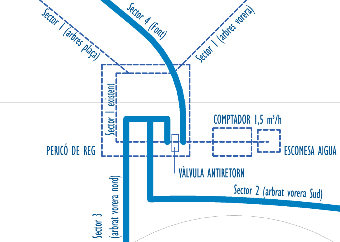
DETALL CAPÇALERA DE REG
