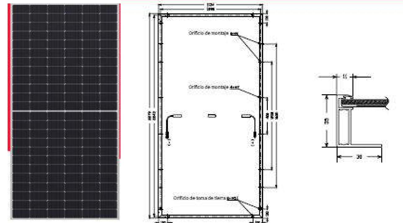
Figura 5: Dimensions del mòdul fotovoltaic proposat
