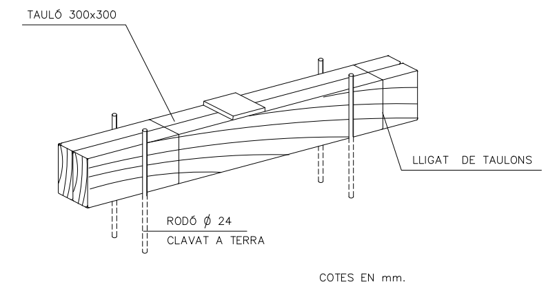
DETALL DE CALZE
